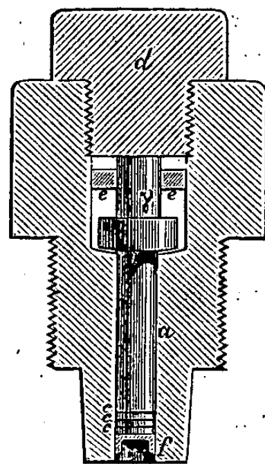
Fig. 1. — Manomètre à écrasement.
