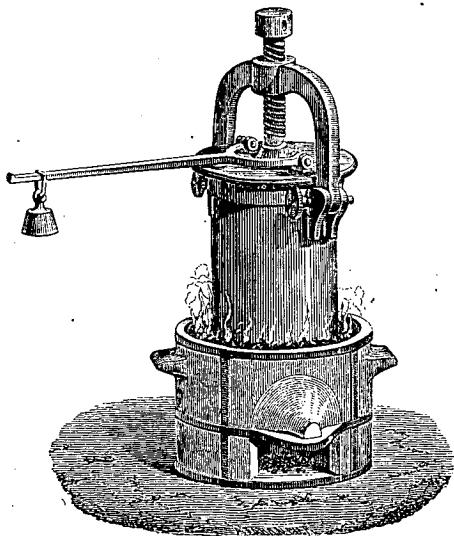
Fig. 70. — Marmite de Papin.
