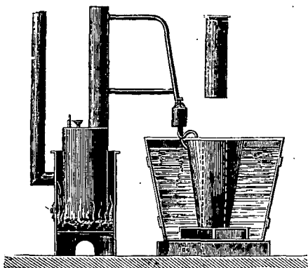
Fig. 88. — Appareil Carré (fabrication de la glace).
