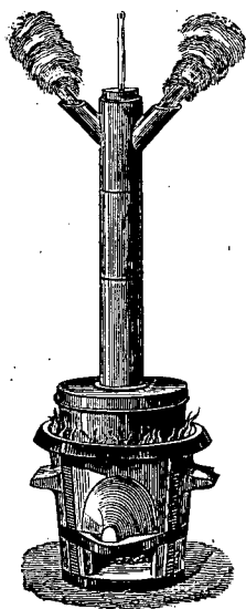
Fig. 8. — Appareil pour marquer le point 100° des thermomètres.
