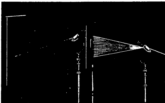
Action d'un prisme sur les rayons simples. (Fig 30)
