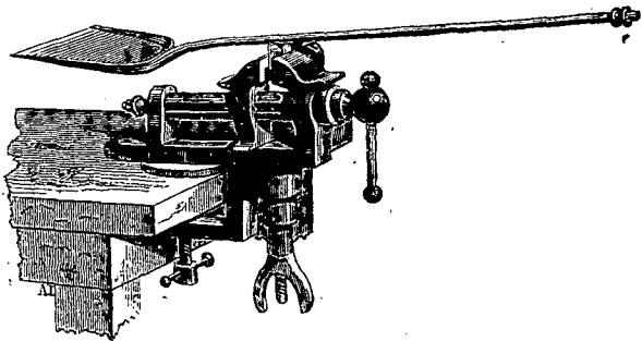
Fig. 56. — Expérience de Trevelyan.
