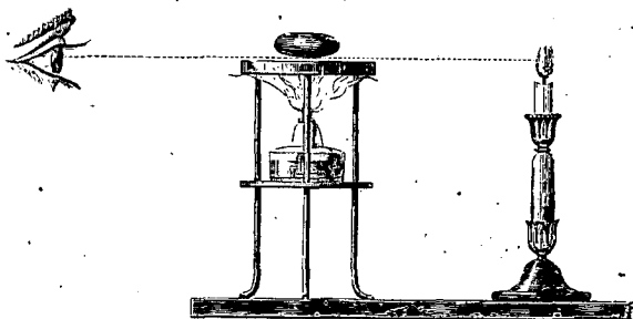
Fig. 78. — Flamme vue entre le globule et la plaque incandescente.
