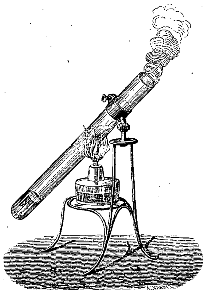
Fig. 44. — Eau bouillant au-dessus de la glace.
