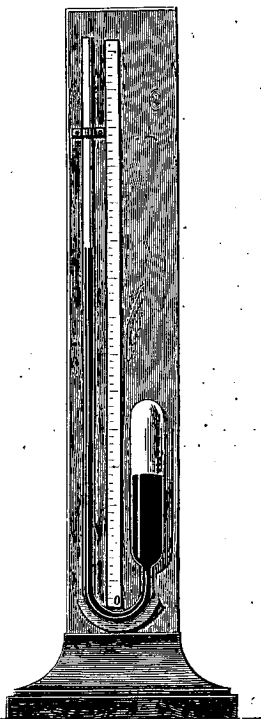
Fig. 81. — Liquéfaction de l'acide sulfureux par la pression.
