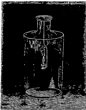
Fig. 12. — Combustion du phosphore dans le chlore.
