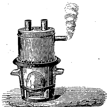
Fig. 37. — Conductibilité du fer et du bismuth.
