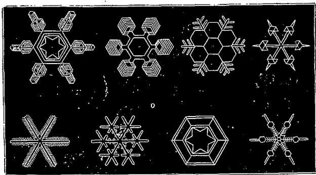
Fig. 60. — Formes diverses de la neige.
