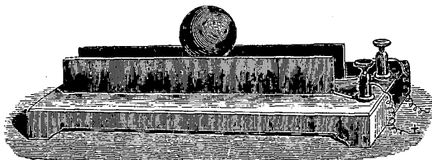
Fig. 57. — Expérience de Gore.
