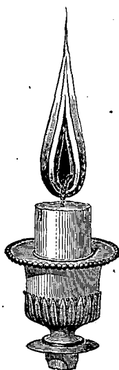
Fig. 15. — Flamme d'une bougie.
