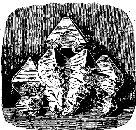
Fig. 91. — Cristallisation d'alun.
