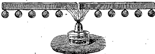
Fig. 55. — Conductibilité des corps solides.
