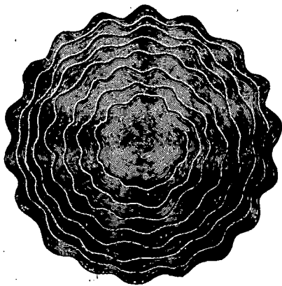
Fig. 77. — Globule à l'état sphéroïdal.
