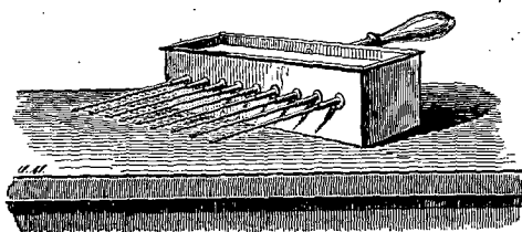
Fig. 36. — Appareil d'Ingenhouz.
