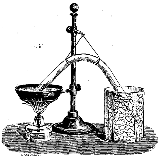
Fig. 82. — Liquéfaction des gaz par le procédé de Faraday et Davy.
