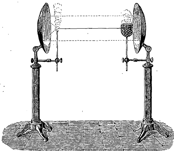
Fig. 24. — Miroirs conjugués.
