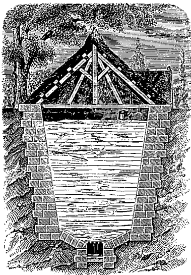
Fig. 41. — Glacière.
