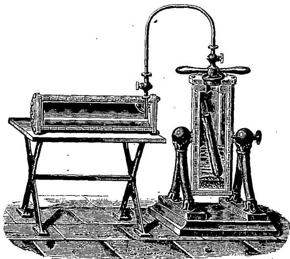
Fig. 85. — Appareil de Thilorier pour liquéfier l'acide carbonique.
