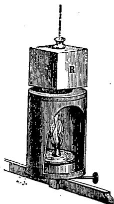
Fig. 52. Cube de Leslie.
