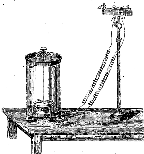
Fig. 5. — Pile et galvanomètre.
