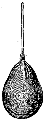
Fig. 49. Dilatation de l'air sous une pression constante.
