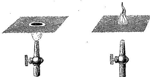
Fig. 50. — Propriété des toiles métalliques.
