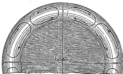
Fig. 48. — Théorie des courants polaires.
