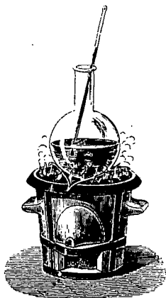
Fig. 58. — Soufre fondant dans un ballon.
