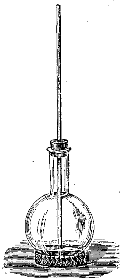
Fig. 51. — Échauffement d'un gaz sous un volume constant.
