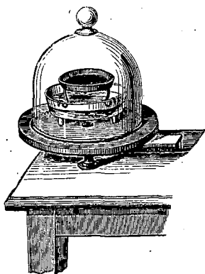
Fig. 86. — Congélation de l'eau par évaporation.
