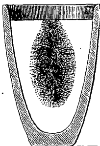
Fig. 59. — Cristallisation du soufre.
