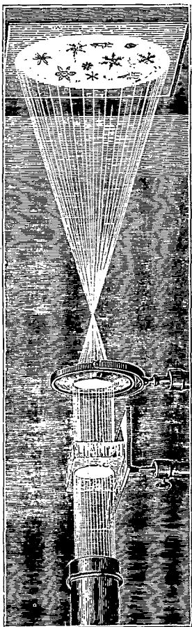
Fig. 65. — Projection des fleurs de la glace.
