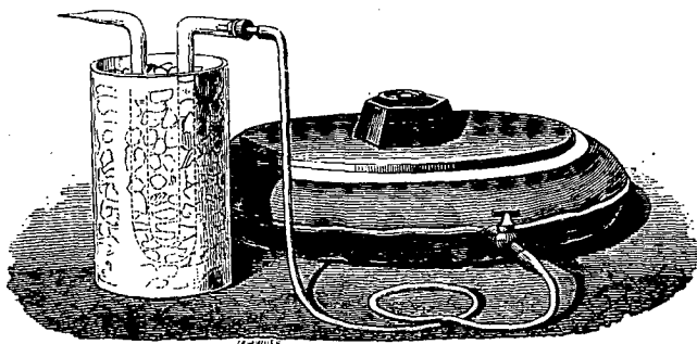
Fig. 80. — Liquéfaction de l'acide sulfureux par le refroidissement.
