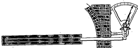
Fig. 10. — Pyromètre de Brongniart.
